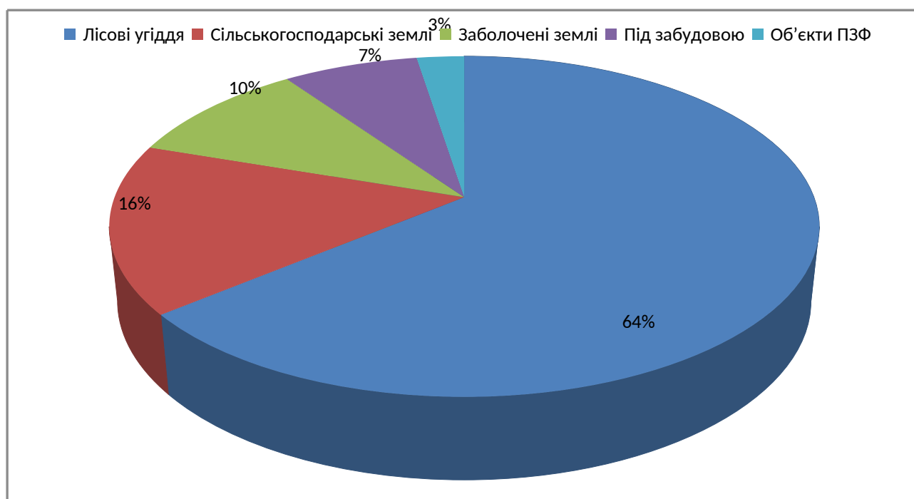
Діаграма 1 Структура земельного фонду Білозірської територіальної громади
